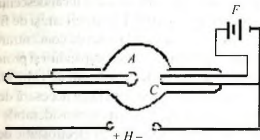
Fig. 1. Tub de raze X: C – catod; A – anod; F – sursă de alimentare a catodului (filament); H – sursă de înaltă tensiune pentru accelerarea electronilor.
