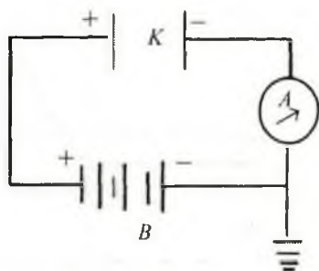
Fig. 21. Schema de conexiune a camerei de ionizare: A – aparat pentru măsurarea intensității curentului; B – baterie; K – cameră de ionizare în formă de condensator plan.
