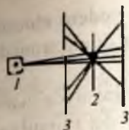
Fig. 16. Schema experimentului lui Rutherford: 1 – sursă de particule \alpha ; 2 – foiță; 3 – ecrane de ZnS.
